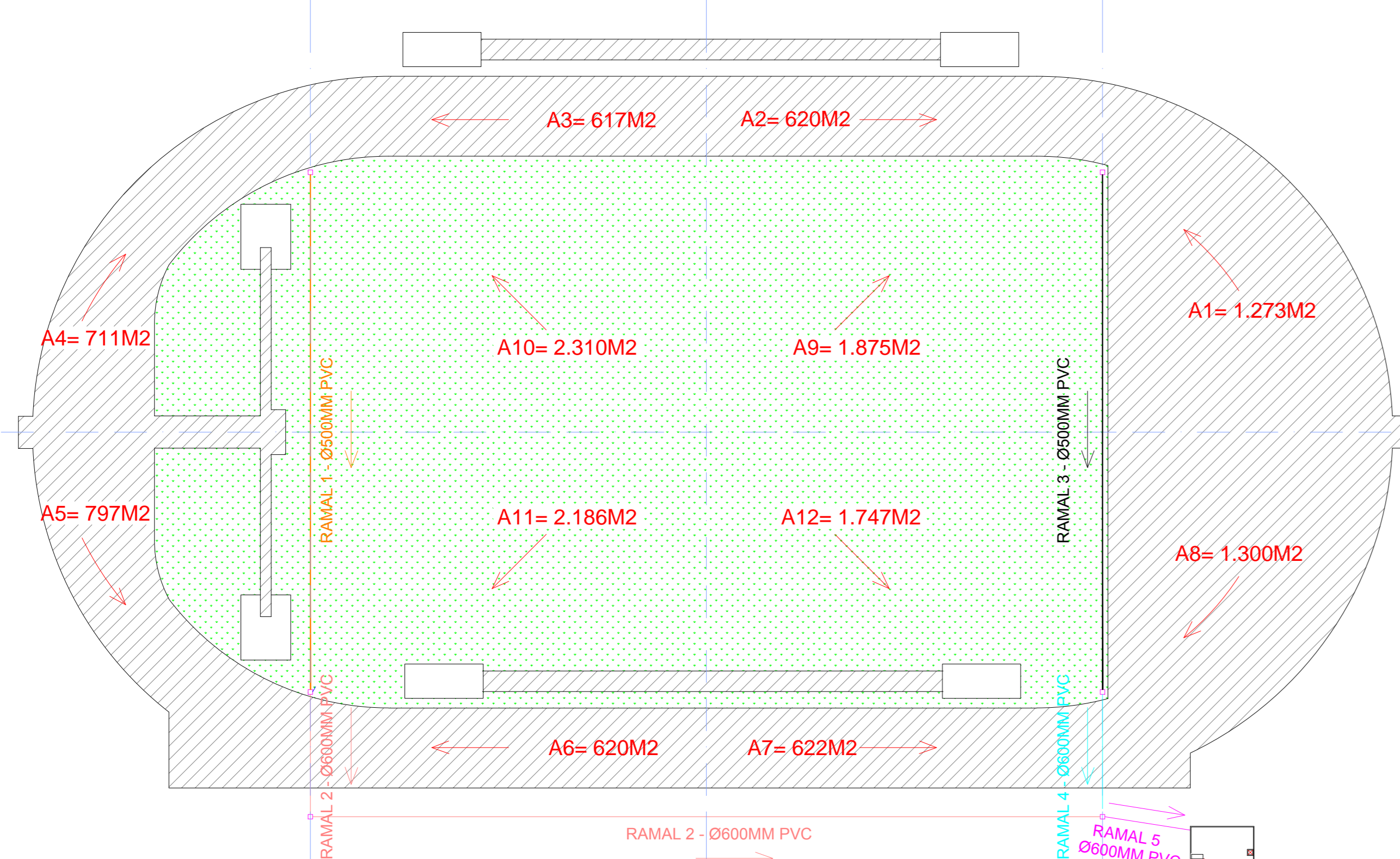
ESQUEMA DRENAGEM UESPI
